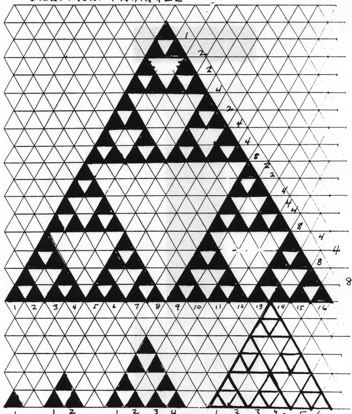
SIERPINSKI TRIANGLE
